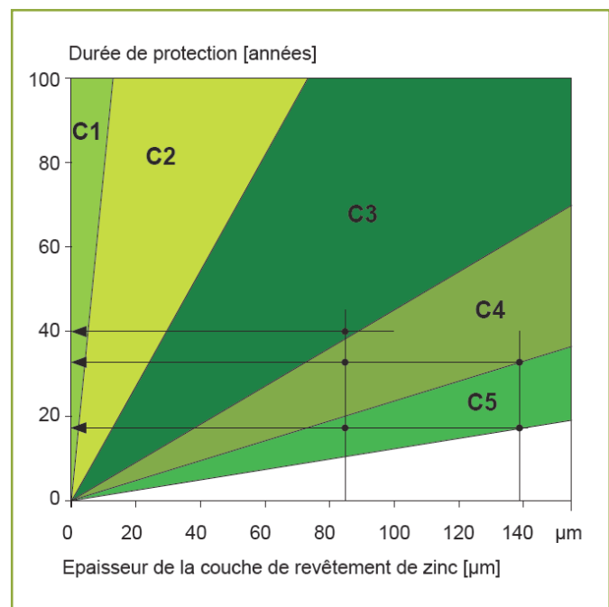
Figure 16 : graphique décrivant l'épaisseur de la couche de revêtement en zinc des aciers galvanisés en fonction du temps.
