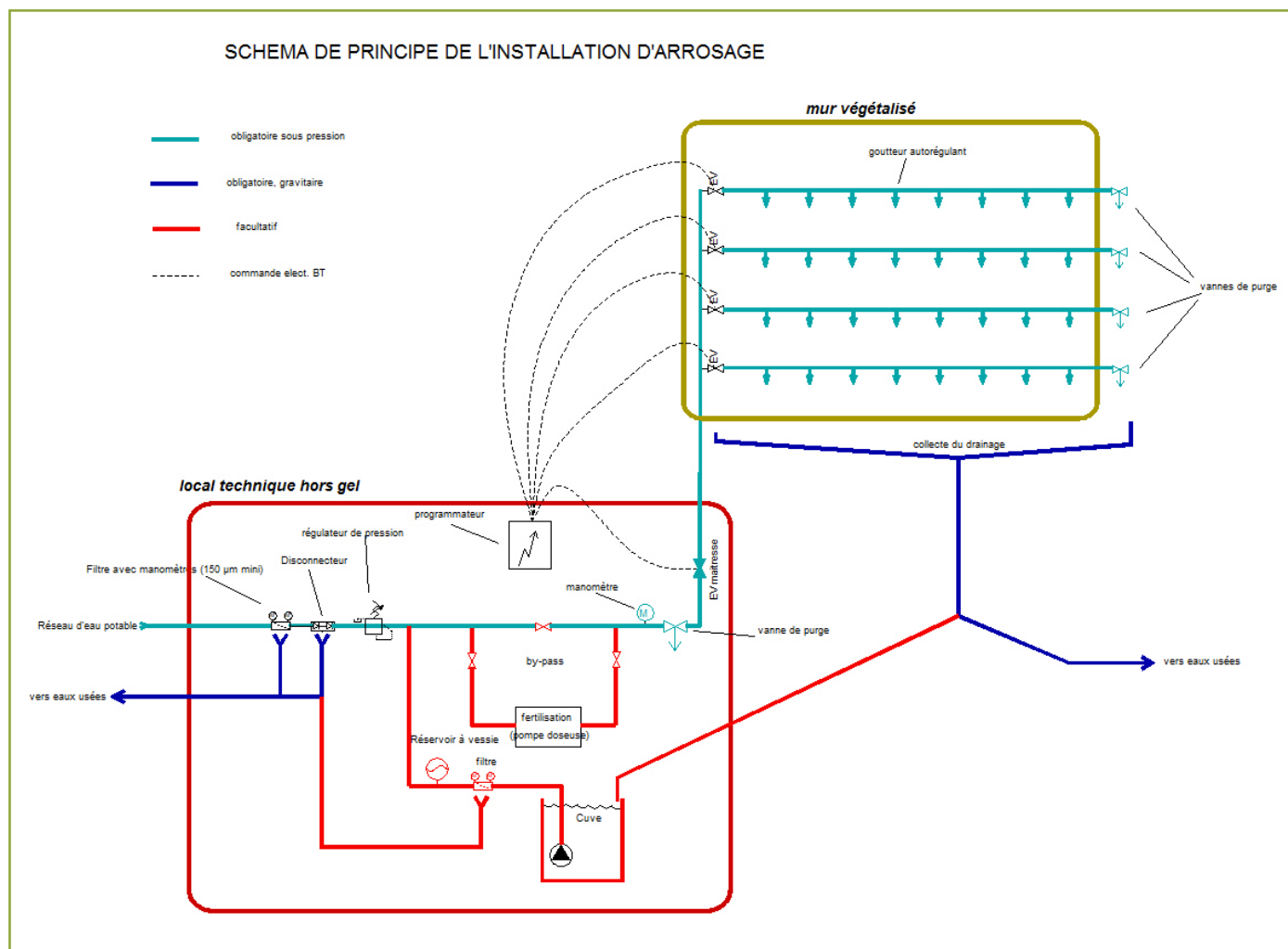
Figure 17 : schéma de principe de l'arrosage des murs végétalisés. Source : P. Faucon.
