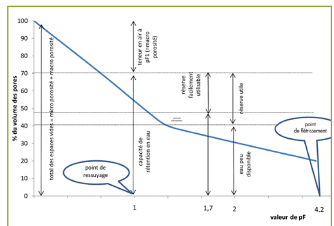
Figure 12 : exemple de schéma des différents degrés de disponibilité en eau en fonction des forces de tension de l'eau dans le sol.
