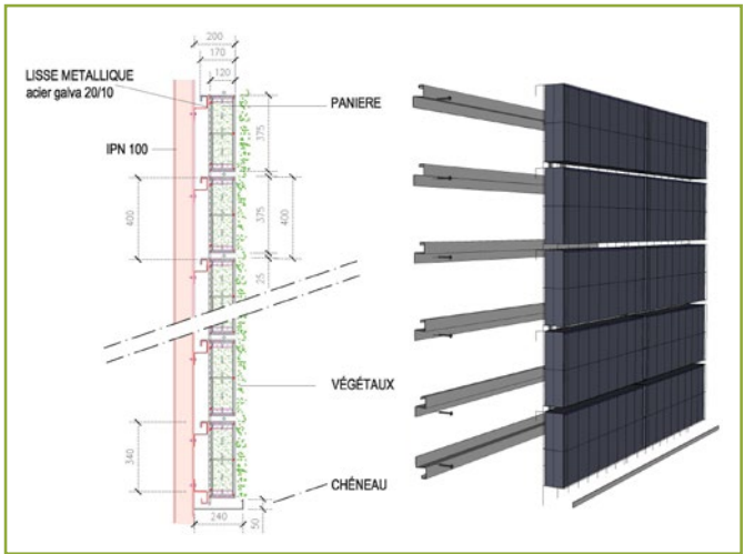
Figure 2 : schémas de végétalisation de façade par gabions. Source : T. Muller.
