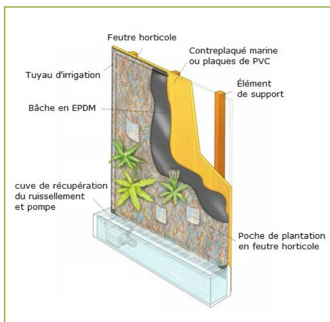
Figure 10 : schéma en coupe d'un mur végétal sur nappe continue. Source : J.-M. Groult.
