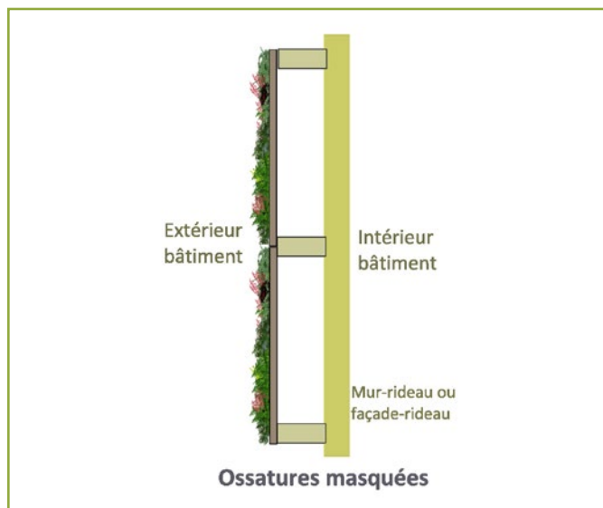
Figure 13 : schéma de mur rideau. Dessin : C. Houel.
