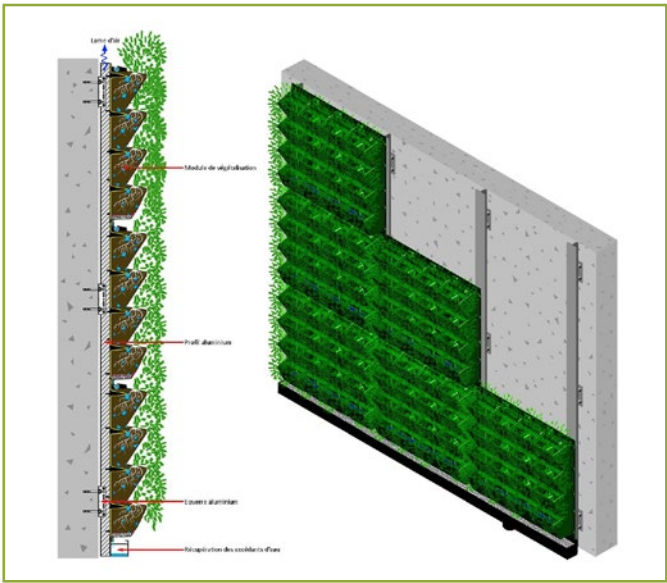
Figure 4 : Schéma d'un exemple de modules préformés. Source : José Dos Santos.
