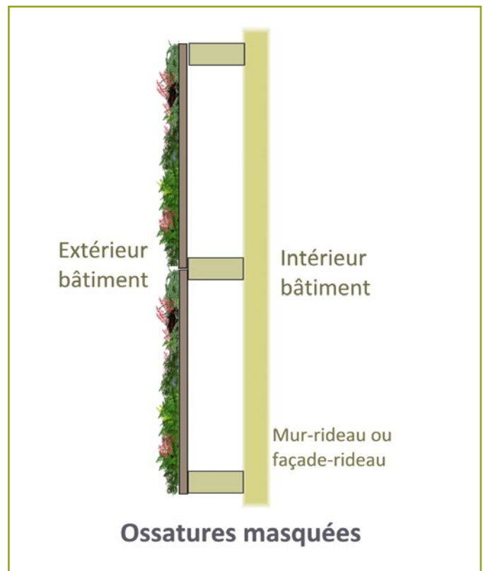
Figure 6 : schéma de mur rideau. Dessin : C. Houel.
