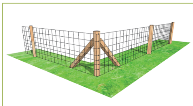
Figure 6. Vue 3D de l'installation d'un grillage noué ou soudé Dessin de C. Houel
