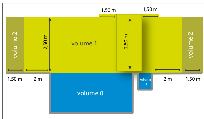
Figure 1: Dimensions des volumes pour piscines et pédiluves
