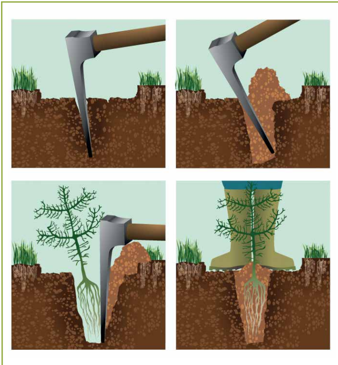
Figure 1 : Plantation en fente d'un plant en racines nues
